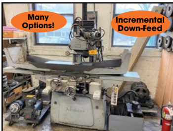
JAKOBSEN 12"x 36" HYD. SURFACE GRINDER
